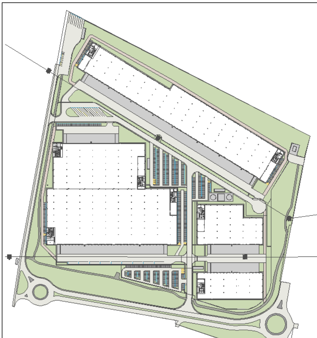
Figura 2: planimetria dello stato di progetto
