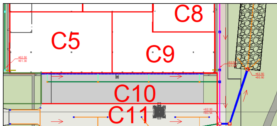
Figura 6: Suddivisione in sottobacini per dimensionamento idraulico tubazioni di collettamento (es. porzione sottobacino C)
